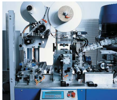
Etikettiermodul (Zubehör)
