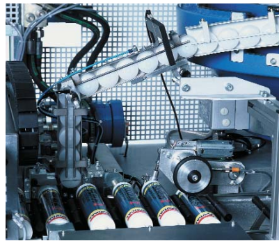
Kolbenetzstation
